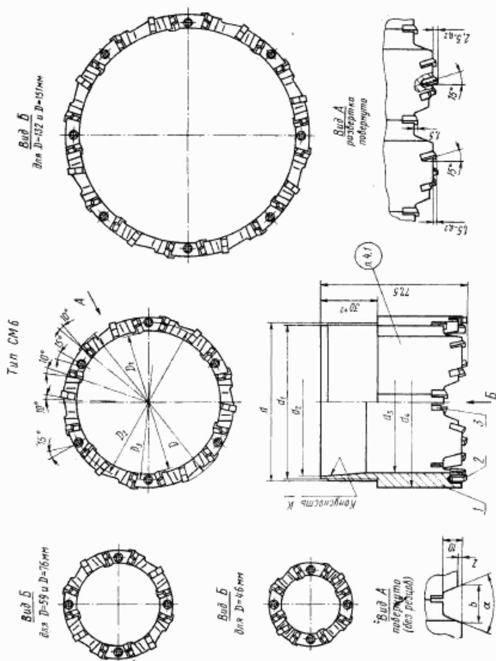
1 - корпус горелки; 2 - пластина твердосплавная Г5106 по ГОСТ 890-67; 3 - вкладыш.
